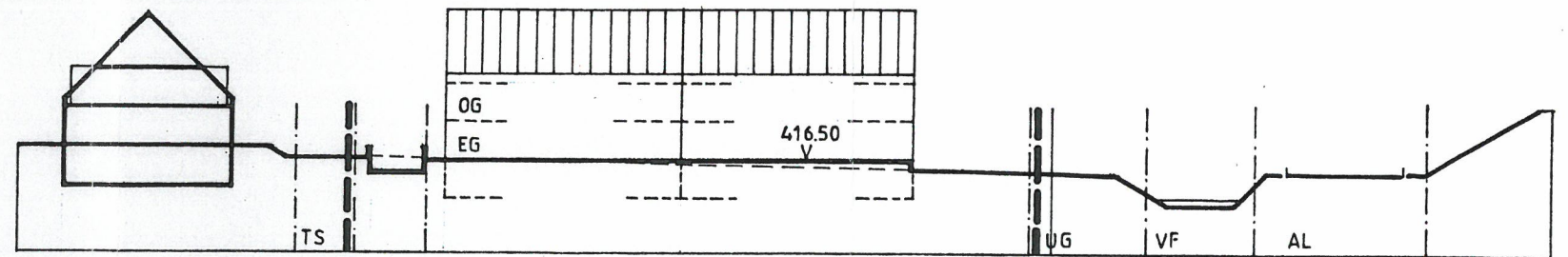
SCHNITT 3
